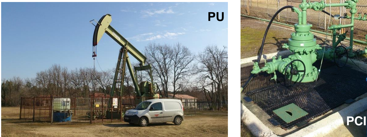
FIGURE 6 : SYSTEMES DE POMPAGES UTILISES
