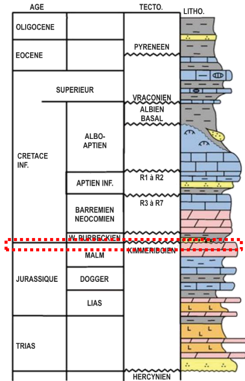
FIGURE 3 : ECHELLE STRATIGRAPHIQUE DU BASSIN AQUITAIN
