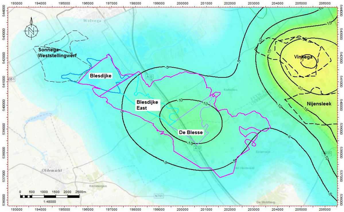
Figuur 15-4 Toekomstige maximale bodemdaling (vanaf 1-1-2018) in millimeters, rondom voorkomen De Blesse - Blesdijke, op basis van modelberekening. Het diepste punt boven de Blesse is minder dan 2 cm (uit ref. 50).
