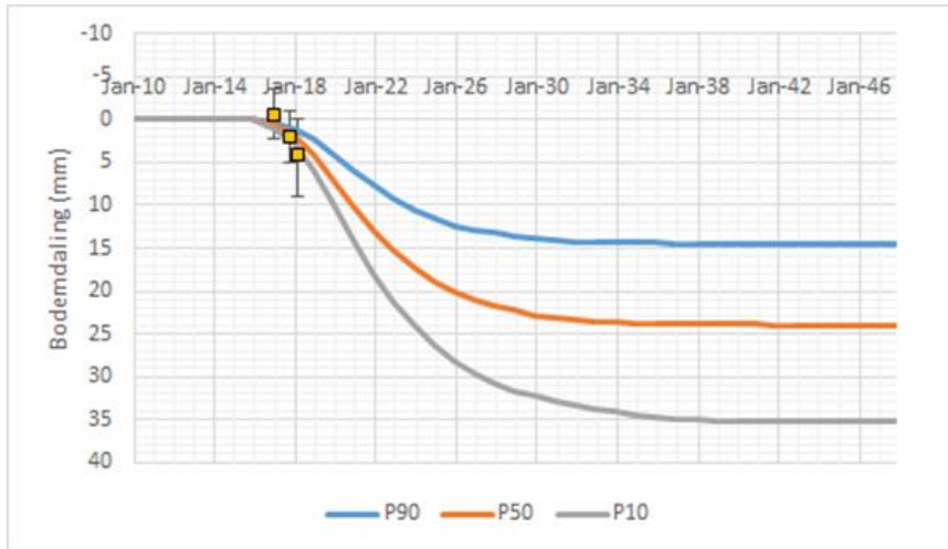
Figuur 16-10 Diever verwachtingskrommen na uit voorzorg aanpassen van het H case depletiegebied.
