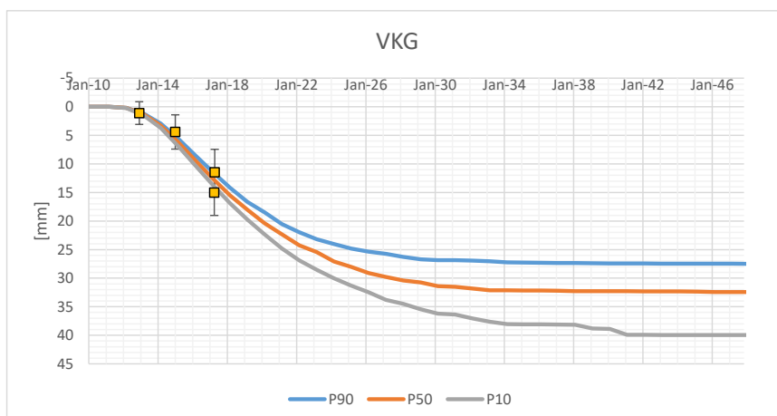
Figuur 16-4 Heralibratie van de Vinkega dalingskrommen aan de metingen (GPS en waterpassing).
