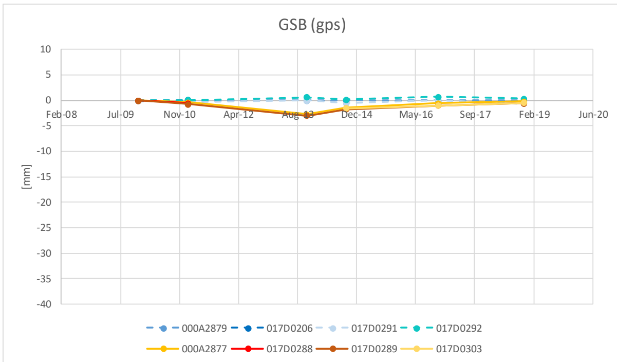
Figuur 18-1 Bodemdaling Geesbrug uit GPS-meting. GSB-punten in oranje, aansluitpunt (Stuifzand) in blauw. Data uit ref. 59). De punten rond Meppen zijn niet getoond, want liggen in het invloedsgebied van de NAM winning Oosterhesselen.
