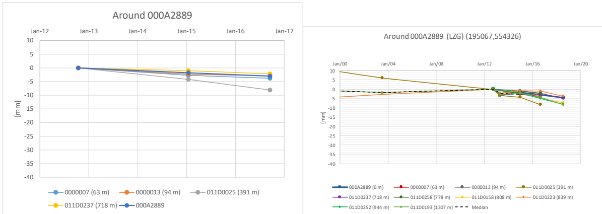
Figuur 13-2 Links: Peilmerk dalingen rond de Langezwaag locatie (000A2889), uit ref. 45. Dalingen van 0.2-0.4 cm worden gemeten, vergelijkbaar met de meetonnauwkeurigheid. (011D0025 lijkt niet stabiel). Data uit ref. 45. Het peilmerk 000A2889 is diep gefundeerd, de anderen niet. De rechtergrafiek geeft dalingen uit de RWS-database (tot iets verder in het verleden).
