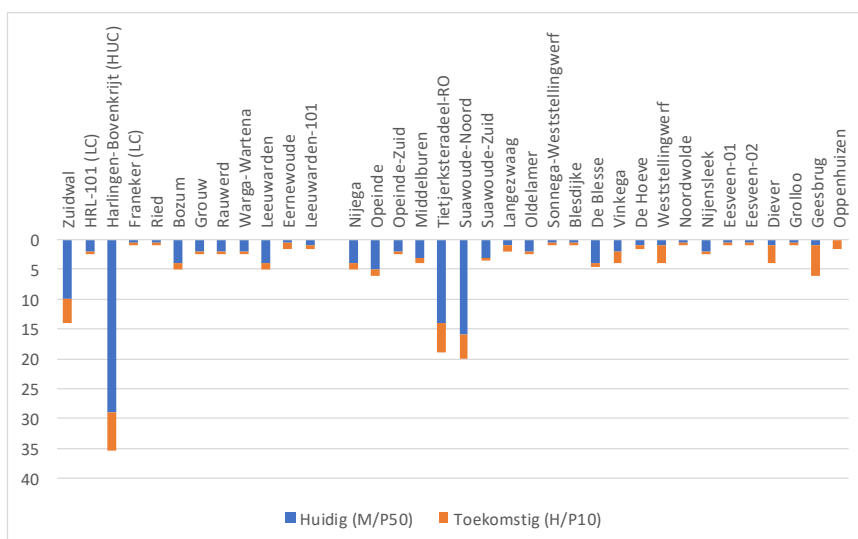
Figuur 3-2 – Grafische weergaven van huidige & uiteindelijke bodemdalingen per voorkomen. Het betreft de daling door winning uit het betreffende voorkomen apart. Waar komen overlappen is de bodemdaling de som van meerdere bijdragen. Die samenstellingseffecten zijn meegenomen in de kaarten, en bij de calibratie met de metingen.
