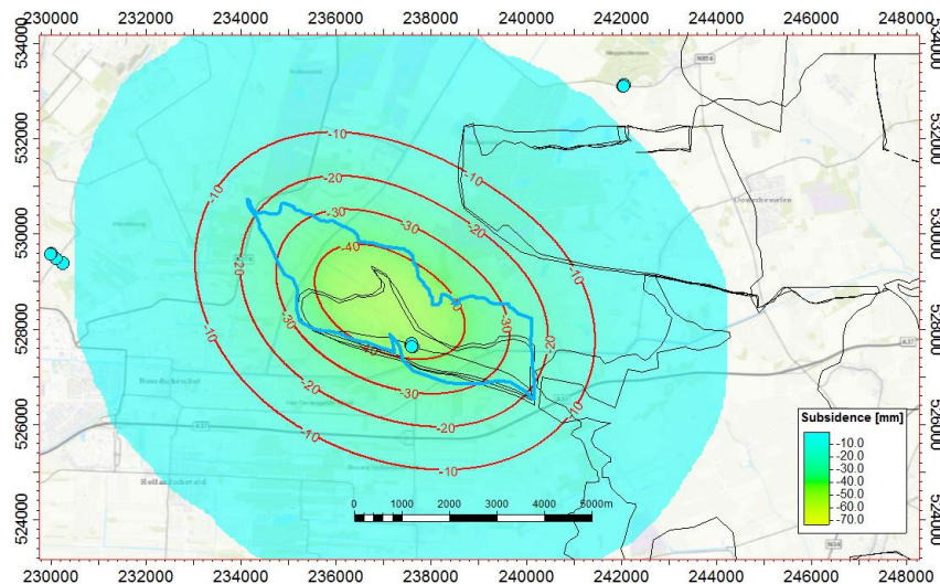
Figuur 18-3 Kaart Geesbrug. De GPS-meetpunten als blauwe cirkels (ref. 59). De verwachte toekomstige daling is weergegeven [mm]. Ten noordoosten van Geesbrug liggen een aantal NAM winningen (o.a. Oosterhesselen). De daling is binnen de verwachting uit het vigerende winningsplan: op de metingen is geen daling zichtbaar.
