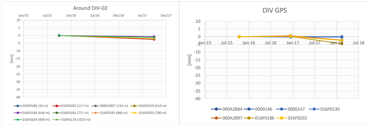
Figuur 16-7 Waterpas- (links) en GPS-data (rechts) bij Diever. Rechts in blauw referentiepunt Boijl, in oranje Diever (ref. 56).
