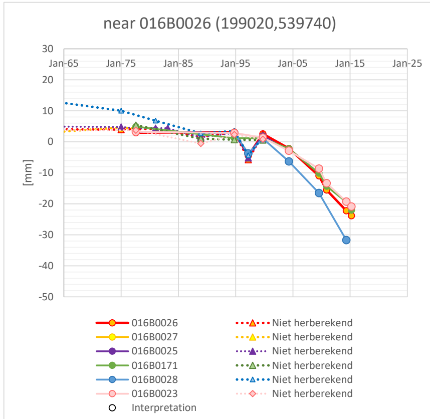
Figuur 15-2 Bodemdaling op hetzelfde punt als hierboven, maar nu uit de RWS-database (ref. 9). Het begin van de gaswinning is duidelijk zichtbaar. Het blauwe punt lijkt als enige ook al daling te vertonen vóór 1999, mogelijk is daar een stabiliteits- issue .
