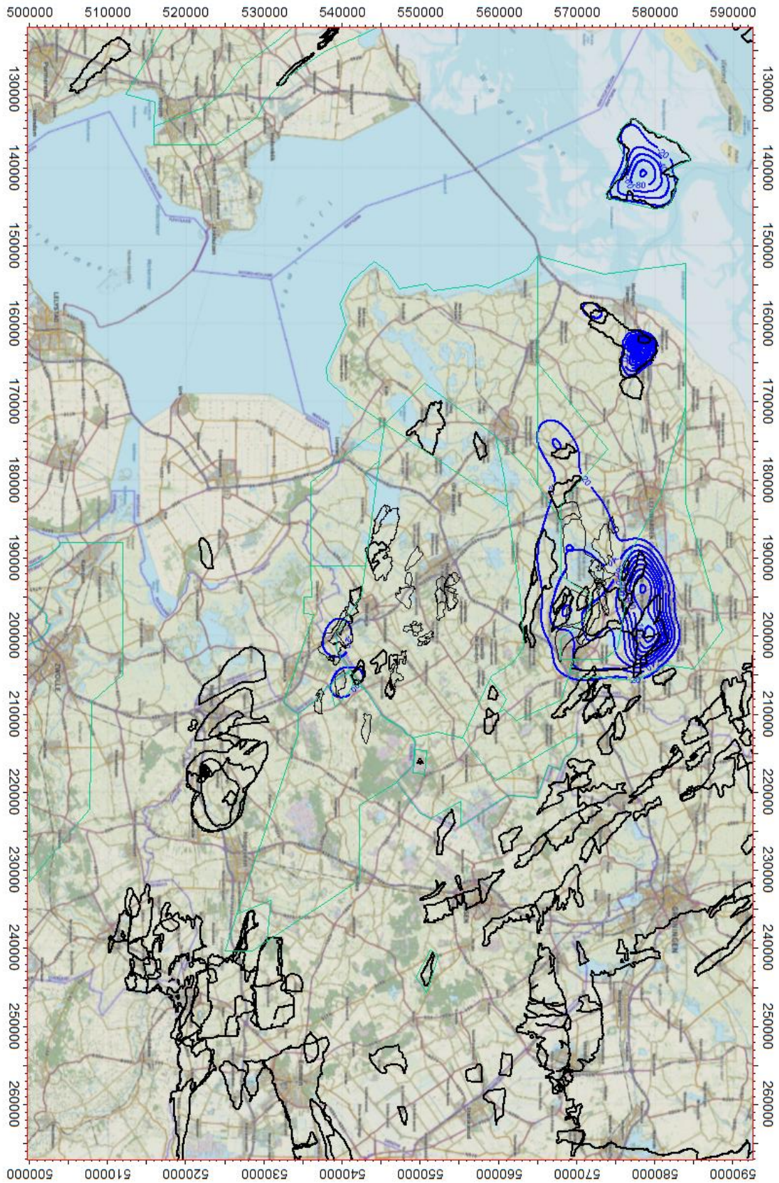
Figuur 3-3 Overzicht geschatte huidige gasbodemdaling (M/P50) door Vermilion gaswinning in Friesland. Overijssel en Drenthe. (Contouren in blauw 20, 40, 60, ... mm) In de bijlagen zijn zoom-in kaarten te vinden. (Bodemdaling is gerekend vanaf het moment dat de gaswinning in het betreffende gebied begon.)
