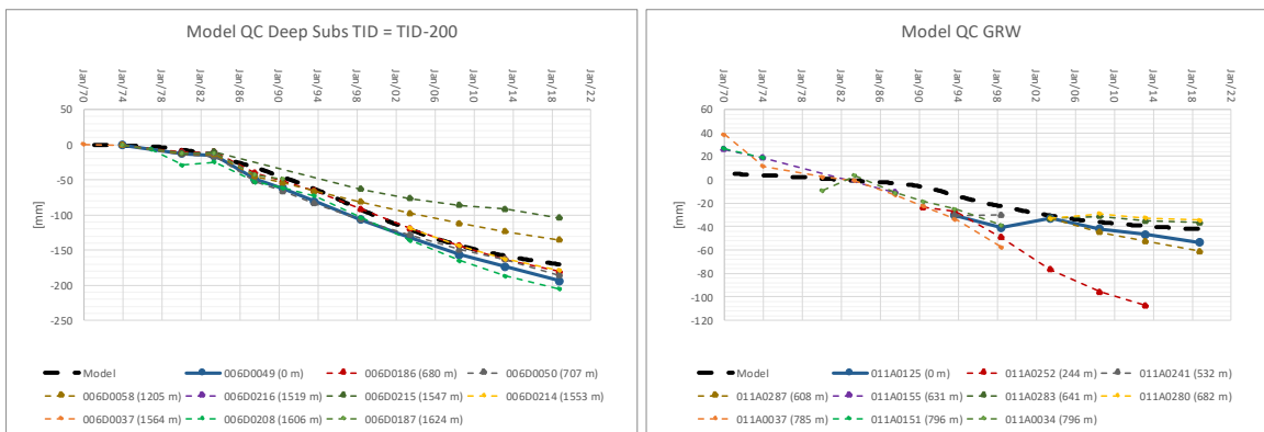
Figuur 12-6 - Voorbeelden van model-calibratie. Links betreft het een punt bij het diepste punt in LEW-O, bij de TID-200 locatie. Rechts gaat het om een punt in het westen van het meetnet, waar autonoom en gasdaling moeilijk helder te scheiden zijn. [Verticale schalen verschillen.]
