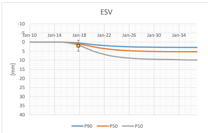
Figuur 16-11 De waterpassing boven het Eesveen voorkomen laat geen significante daling zien, maar dat was ook niet verwacht. De verwachting wordt dus niet aangepast.
