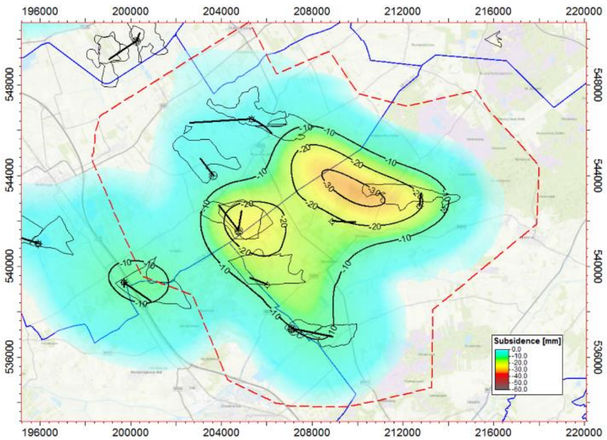
Figuur 16-13 Op basis van aan de metingen gecalibreerde modellen geschatte toekomstige daling [mm]. De begrenzing van het meetplan is met een rode stippellijn aangegeven.
