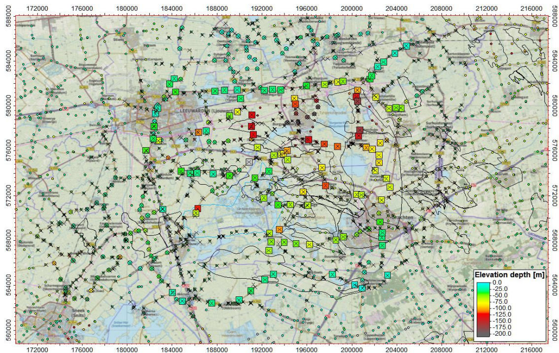
Figuur 12-7 Overzicht van de dalingsmetingen in het Leeuwarden-Oost gebied, mm. RWS-data als kleine cirkels, data uit het meetplan Leeuwarden-Oost/Oosterend als vierkanten waar geldig 1970-2018. Kruisjes geven de punten uit het meetplan waar geen data over de volle periode (1970-2018) beschikbaar is.
