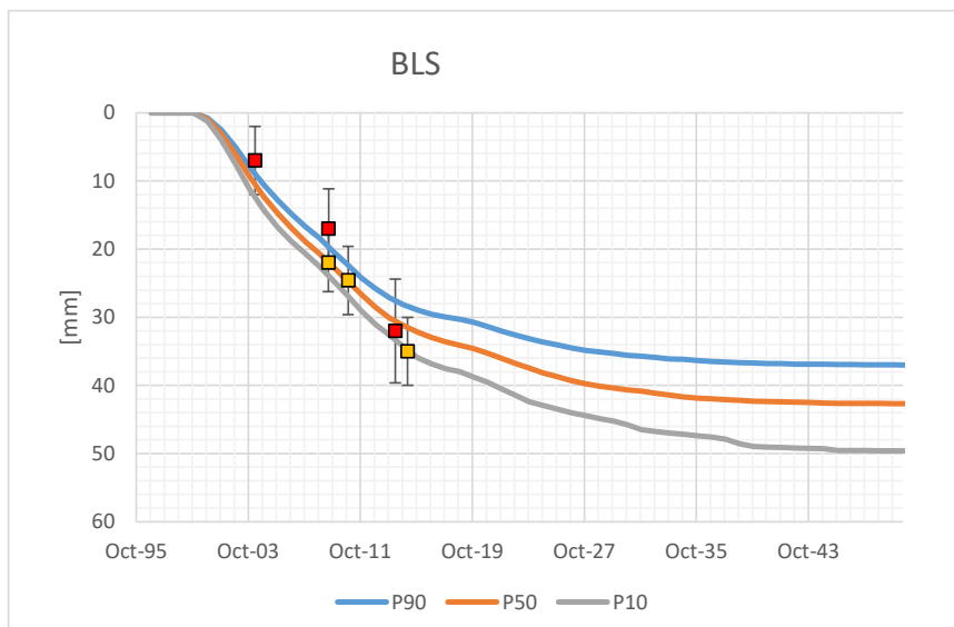
Figuur 15-3 Gecalibreerde dalingsverwachting van BLS in het diepste punt, gecalibreerd aan de metingen. Hier zijn punten, gededuceerd uit de RWS/NAP-database, toegevoegd in rood. (Uit ref. 50). Merk op dat het punt waar de diepste toekomstige daling wordt verwacht niet precies samenvalt met het punt waar de diepste historische daling is.
