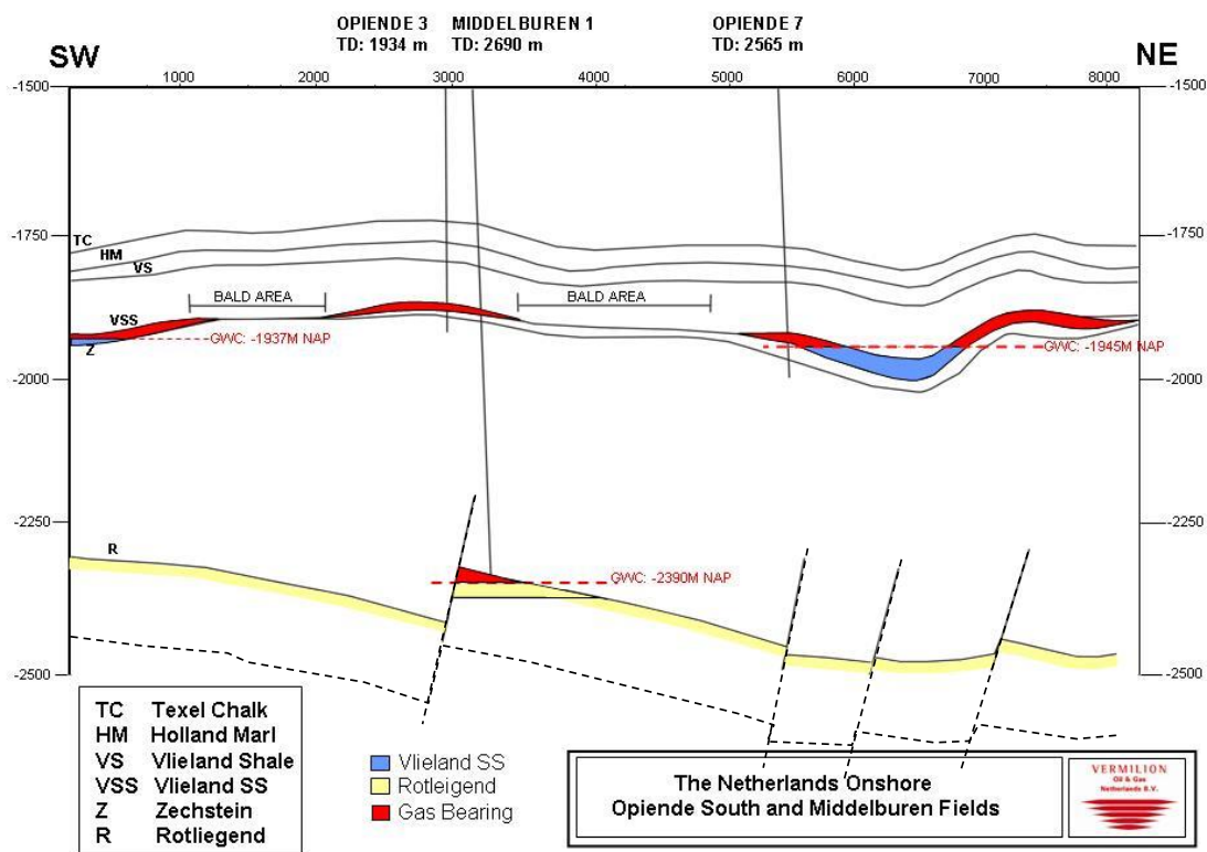
Figuur 12-1: Geologische doorsnede door de voorkomens Opiende-Zuid en Middelburen als illustratie van de boven elkaar liggende gasvoerende zones in het Leeuwarden-Oost gebied. De begrenzingen tussen de velden in de Vlieland formatie zijn gebieden waar de zanddikte nul is ("bald area"). Ook is te zien dat de Rotliegend voorkomens alleen in het bovenste stukje gasvoerend zijn. De uitzonderingen zijn in dit opzicht alleen TID en SUW-N.
