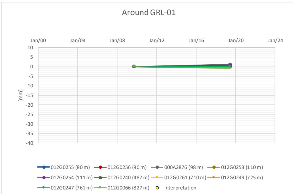
Figuur 17-1 Peilmerkgedrag uit waterpassing 2019, rond de locatie van GRL-01 (ref. 57). Daling is net waarneembaar.
