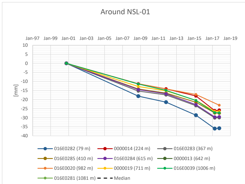
Figuur 16-3 Waterpassingsresultaten bij de NSL-01 oppervlaktelocatie, ten zuiden van Vinkega. De daling na 2011 is het gevolg van winning uit Vinkega (zie tekst).
