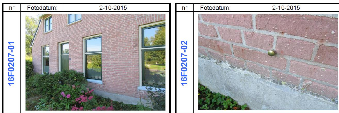
Figuur 2-8 Voorbeeld van een peilmerk (koperen bout) aan een huis. De foto rechts is ingezoomd t.o.v. de linker foto.
