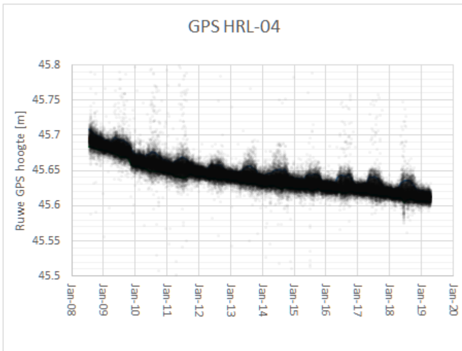
Figuur 10-6 Grafische weergave van de GPS-metingen bij de putlocatie HRL-04. De zwarte puntjes zijn de meetdata. Gezien de (seizoensafhankelijke) ruis in de data, is voor de interpretatie de mediaan-gefilterde data gebruikt (“P50”).
