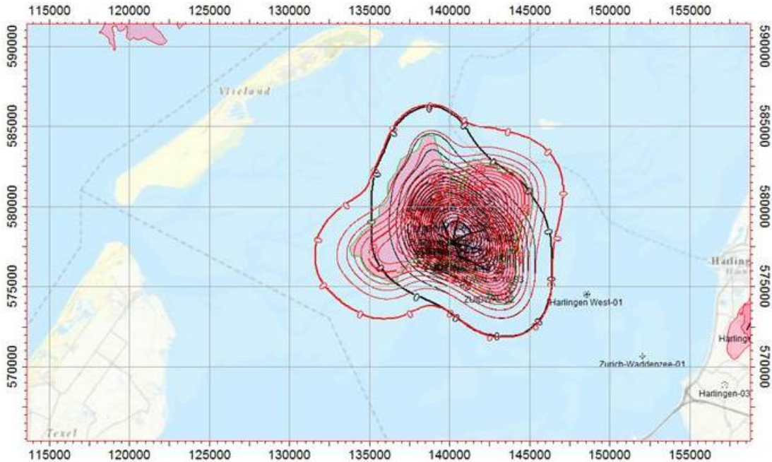
Figuur 9-3: Verwachte eindsituatie van de bodemdaling, in relatie tot het vasteland van Friesland en Vlieland. De bodemdalingsskom is beperkt tot de Waddenzee. Er zijn twee kommen getekend (in rood en zwart) die de onzekerheid over de grootte van het depletiegebied weergeven. Voor de komvolume berekeningen wordt de rode kom gebruikt (ref. 23, 24).
