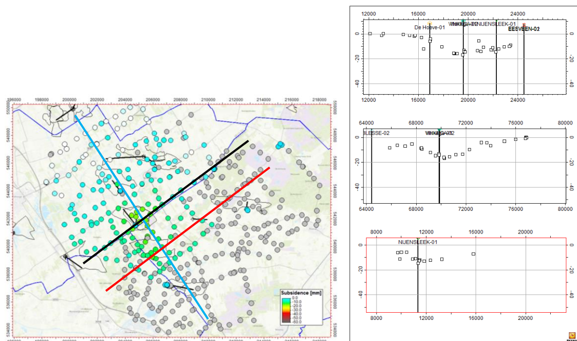
Figuur 16-5 Bodemdaling 2011-2017 in mm, voor dat deel van de meetplannen waar in die jaren een meting is gedaan. Overige punten in grijs. Drie cross-secties (sterk verticaal uitvergroot, verticaal in mm; van boven naar beneden: blauw NW→ZO, zwart, rood ZW→NO. Een duidelijke kom is boven Vinkega en Nijensleek te zien. In deze periode produceerde Vinkega (vanaf 2011) en Eesveen & Diever (vanaf 2015). Omdat Nijensleek niet produceerde in deze periode (gestopt in 2006) is het waargenomen effect het gevolg van gaswinning uit Vinkega.
