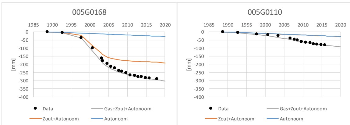
Figuur 10-5 Resultaten van 2018 op dezelfde punten als in Figuur 10-4. Links in Herbaijum, rechts bij Franeker. Daling is grafisch opgesplitst naar gas, zout, autonoom.
