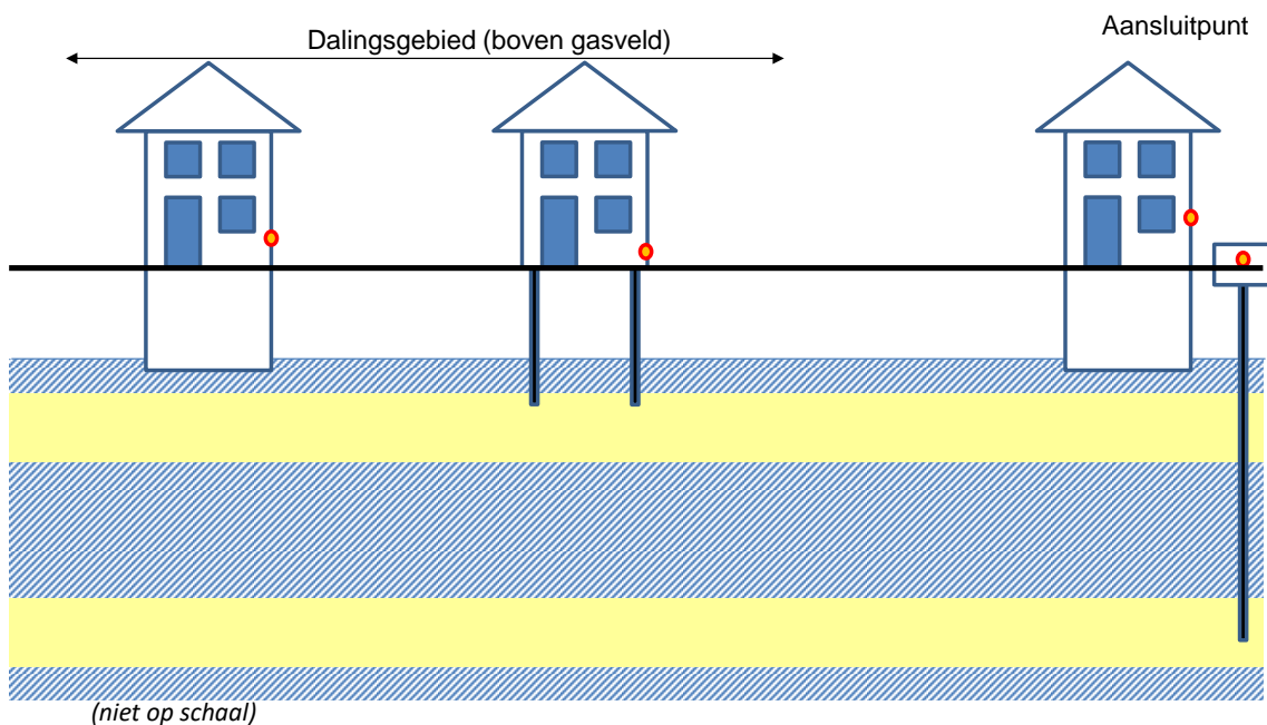
Figuur 2-7 Schematische weergave van peilmerken bij een dalingsmeting. Peilmerken zijn bevestigd aan gebouwen, die op verschillende manieren gefundeerd zijn. De meting wordt uitgevoerd t.o.v. een peilmerk buiten het invloedsgebied van de mijnbouw. Zo 'n aansluitpunt kan diep of ondiep gefundeerd zijn (daar moet bij de analyse rekening mee gehouden worden). Als we de twee rechter meetpunten vergelijken, zien we dat de meest rechtse dieper gefundeerd is. Dit meetpunt is ongevoelig voor inklinking van de lagen boven de funderingsdiepte. (Vgl. ref. 3, fig. 10)
