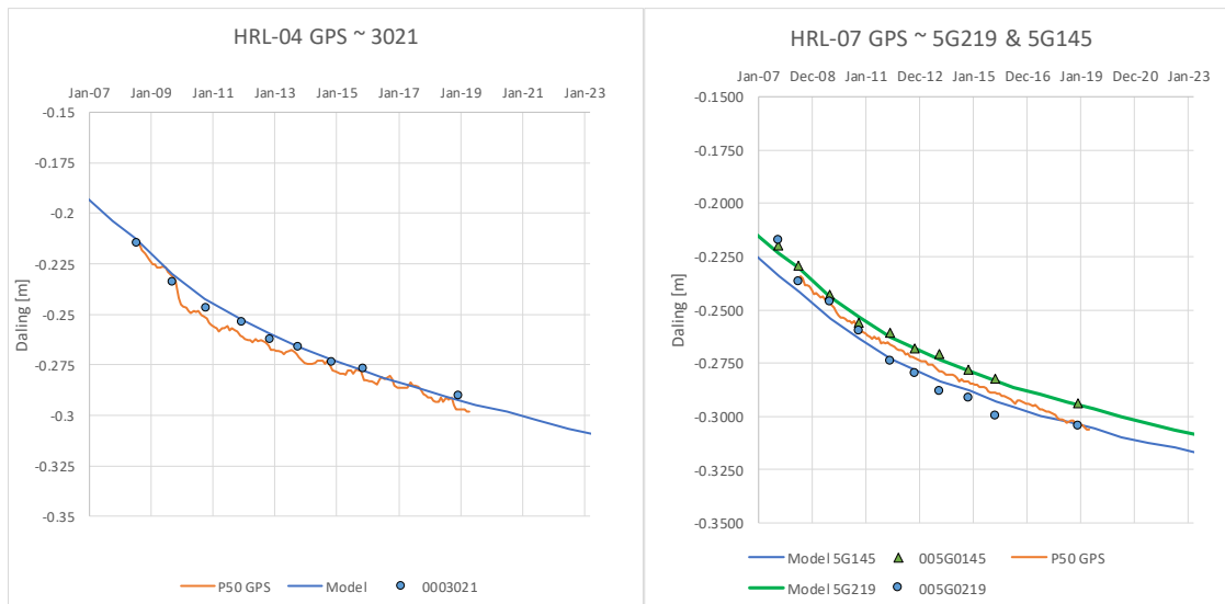
Figuur 10-7 Vergelijking van de permanente GPS-metingen met de modellen. Getoond wordt de mediaan-gefilterde GPS-data ("P50"), en de waterpassingen die nabij die punten zijn uitgevoerd. Bij HRL-07 is er een gradiënt in de bodemdaling, en daarom zijn twee punten (en hun model-curves) als referentie genomen.
