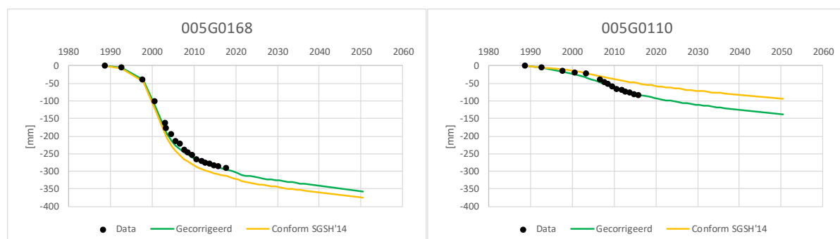
Figuur 10-4 Illustratie van de impact van de correctie aan de hand van twee peilmerken. Links in Herbaijum, rechts bij Franeker. Het SGSH model in oranje, de correctie in groen, waterpasdata in blauw. (Figuur uit ref. 20.)
