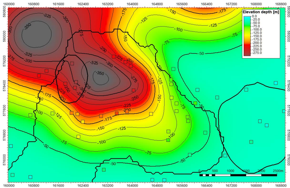
Figuur 10-8 Kaart van totale bodemdaling 1988-2015, in mm. Getoond is de modeldaling, en de metingen die data 1988-2018 hebben (driehoeken). Voor de calibratie moeten alle oorzaken meegenomen worden: zout, gas en autonoom, en dat totaal is dan ook wat de kaart laat zien. Contourinterval 25 mm.
