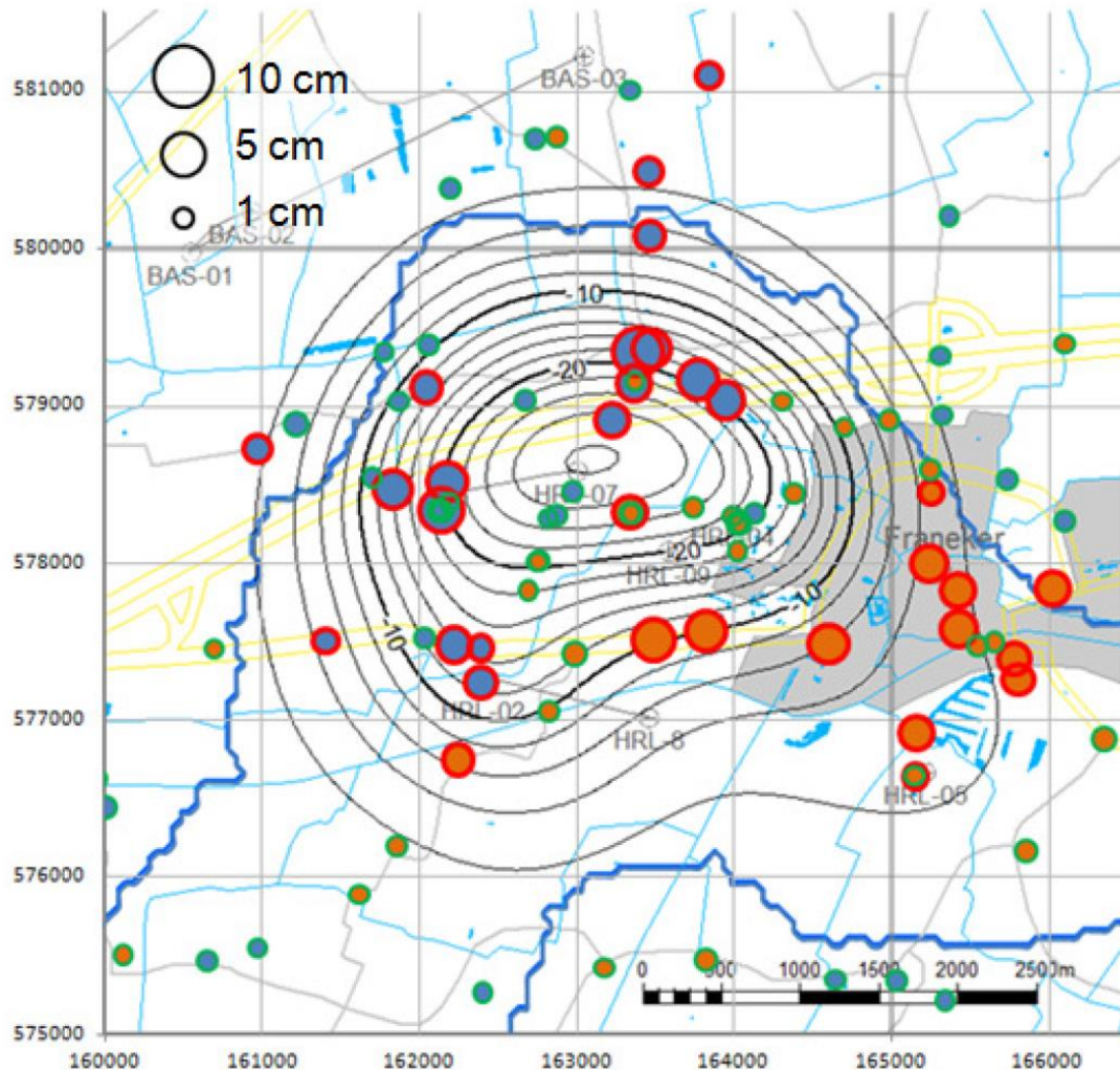
Figuur 10-3 Door SGSH opgemerkte discrepanties tussen model en metingen (blauw: te veel daling in model oranje: te weinig daling in model). Dit is Figuur 6.8 uit ref. 32. Het blauwe polygon geeft de contour van het Harlingen-Bovenkrijt voorkomen aan; de zoutwinningslocaties (BAS-01, BAS-02 en BAS-03) zijn ook te zien ten noordwesten van het gasvoorkomen.
