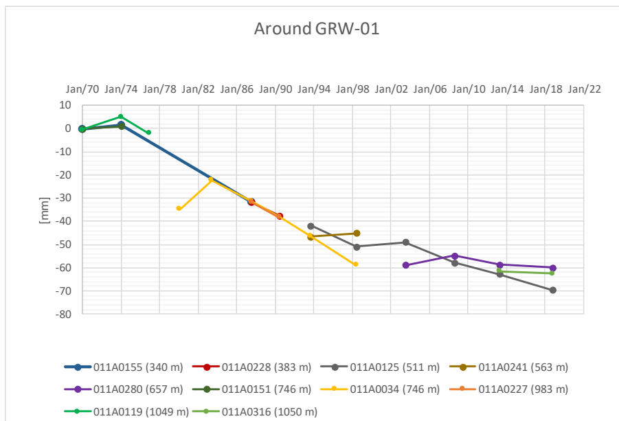
Figuur 2-11 Voorbeeld van een locatie waar de peilmerken in de buurt steeds over een ander tijdsinterval actief waren. Op dit moment zijn nog drie van de peilmerken actief.
