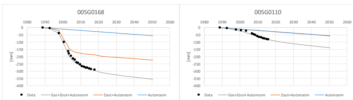
Figuur 10-11 Bodemdalingvooruitzichten op de peilmerken van Figuur 10-5. Links in Herbaijum, rechts bij Franeker. De toekomstige zoutdaling wordt verwaarloosbaar geschat op deze locaties.
