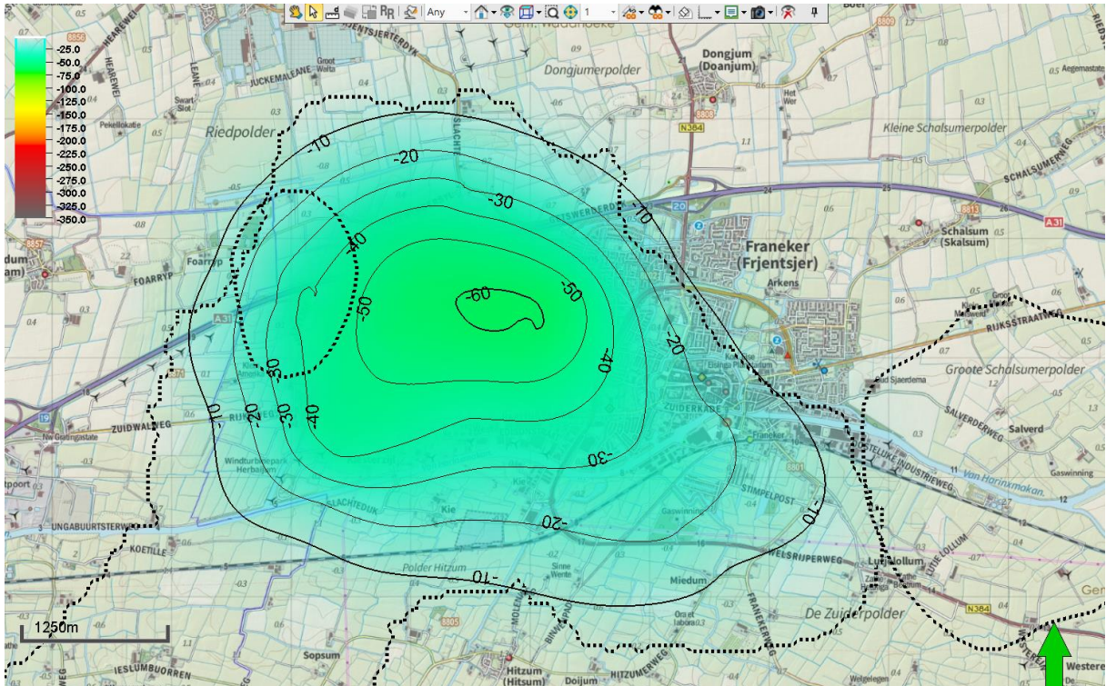
Figuur 10-15 Gasdaling 2018-2050, in mm. Op het diepste punt wordt nog ~6 cm gasdaling verwacht. Contourinterval 10 mm.
