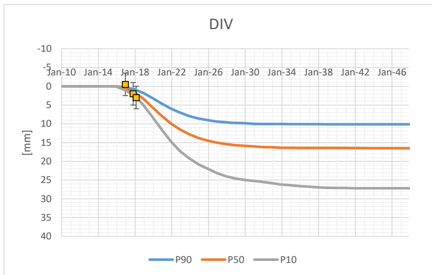
Figuur 16-8 Heralibratie van de Diever dalingskrommen aan de metingen (GPS en waterpassing). De resultaten leiden tot een lichte verhoging van de P10, maar de vorige P10-P90-range en deze overlappen grotendeels (ref. 52).
