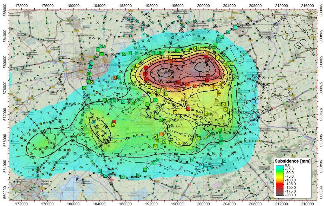
Figuur 12-8 Overzicht van de geschatte gasdaling 1970-2018 in het Leeuwarden-Oost gebied door gaswinningen van Vermilion, mm. Vermilion metingen als vierkanten, RWS-data als kleine cirkels; contouren in blauw 20, 40, 60... mm. De NAM-voorkomens Ureterp, Marum, etc., zijn niet meegenomen; daarom is er geen overeenstemming te verwachten aan de oostrand van het getoonde gebied (ruwweg ten oosten van de lijn X-RD = 202000).
