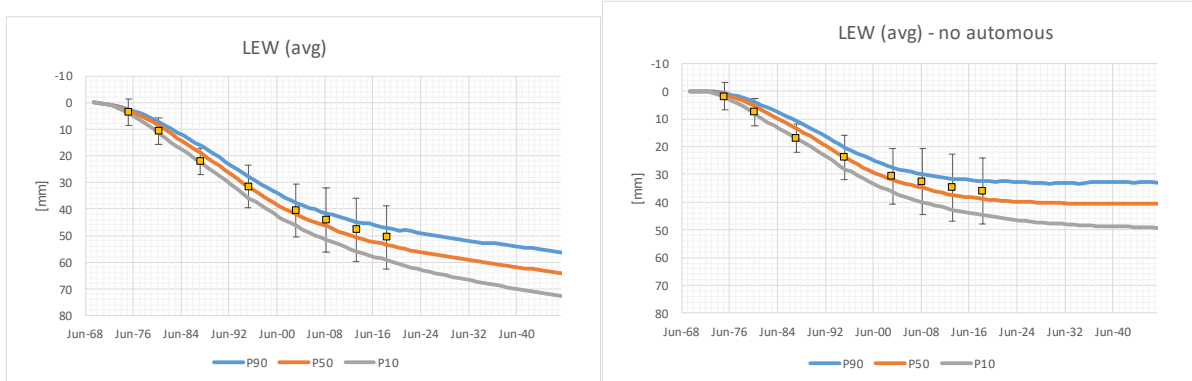
Figuur 12-9 Links: gemeten (gemiddelde over voorkomen) en berekende totale bodemdaling voor het Leeuwarden (LEW) voorkomen, bij voortzetting van de (dalende) productie vanuit het huidige depletiegebied. Er is rekening gehouden met autonome daling (zie tekst), de rechtergrafiek geeft de geschatte gasdaling. Het overgrote deel van de toekomstige gasdaling is na-ijldaling t.g.v. gasproductie uit het verleden. Daling in mm.
