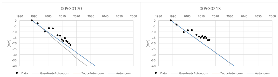
Figuur 10-9 – Vergelijking modeldata met metingen bij het gasvoorkomen Ried (links: westelijke flank RID; rechts: bij de RID-02 locatie). De gemeten daling is ~ 2 cm vanaf 1988, die binnen de bandbreedte van de autonome daling valt. In de westflank is de invloed van HUC te zien.
