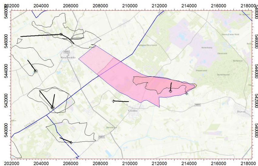
Figuur 16-9 Naar analogie met Vinkega, wordt voor Diever uit voorzorg een mogelijk vergroot depletiegebied als H case aangenomen. Er is geen indicatie in de dalingsmetingen, daarin is geen komvorm te zien. De vorm van het gebied volgt de Rotliegend breukstructuur. Toepassing van deze H case leidt tot een P10 uiteindelijke bodemdaling van 3.6 cm.
