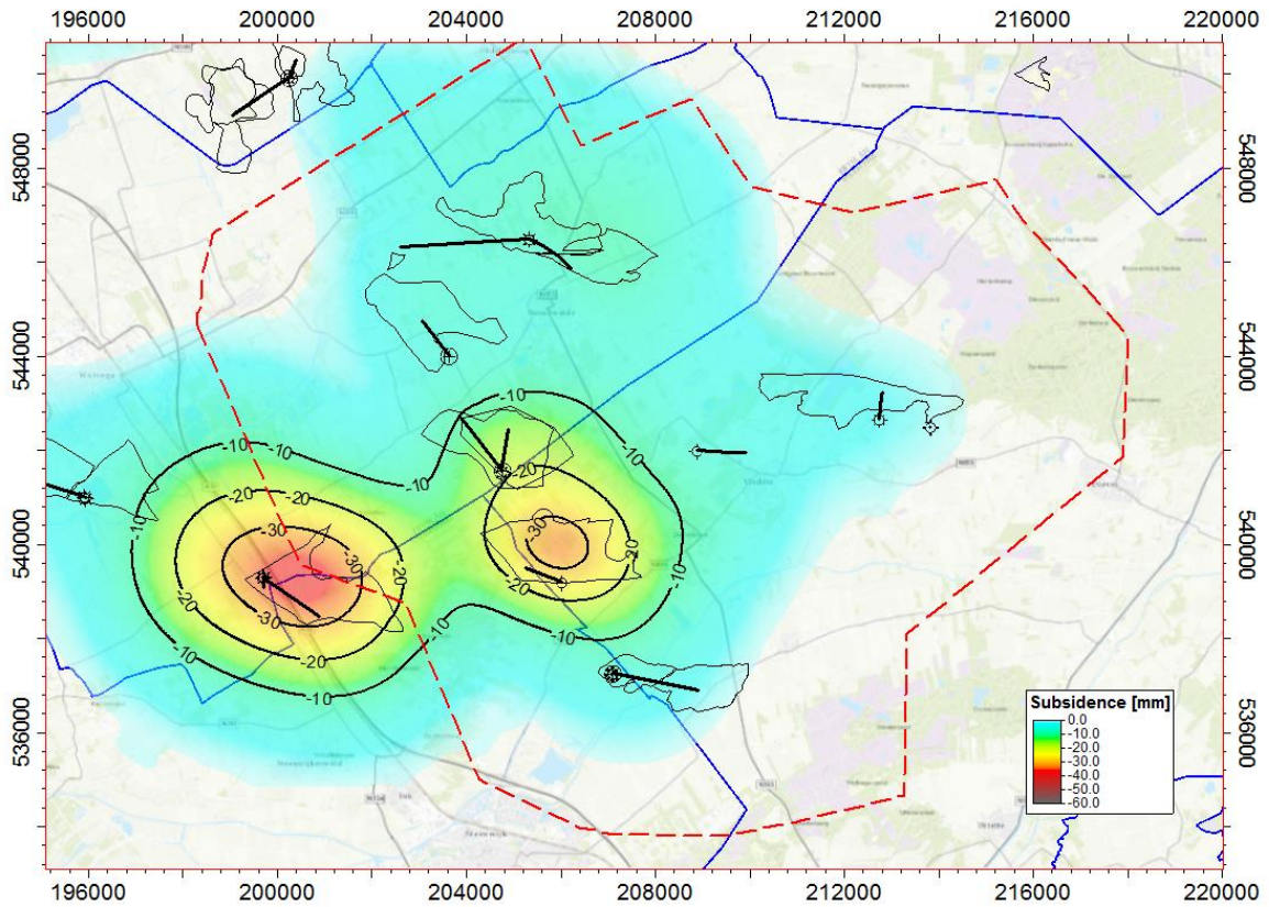
Figuur 16-12 Op basis van aan de metingen gecalibreerde modellen geschatte huidige daling door gaswinning [mm]. De begrenzing van het meetplan is met een rode stippellijn aangegeven.
