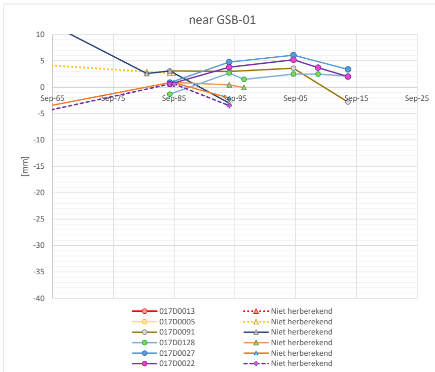
Figuur 18-2 Peilmerkgedrag uit RWS-database rond de locatie van GSB-01 (ref. 9). Er is niet significant meer daling na 2009 dan daarvoor. (De winning begon in 2009)
