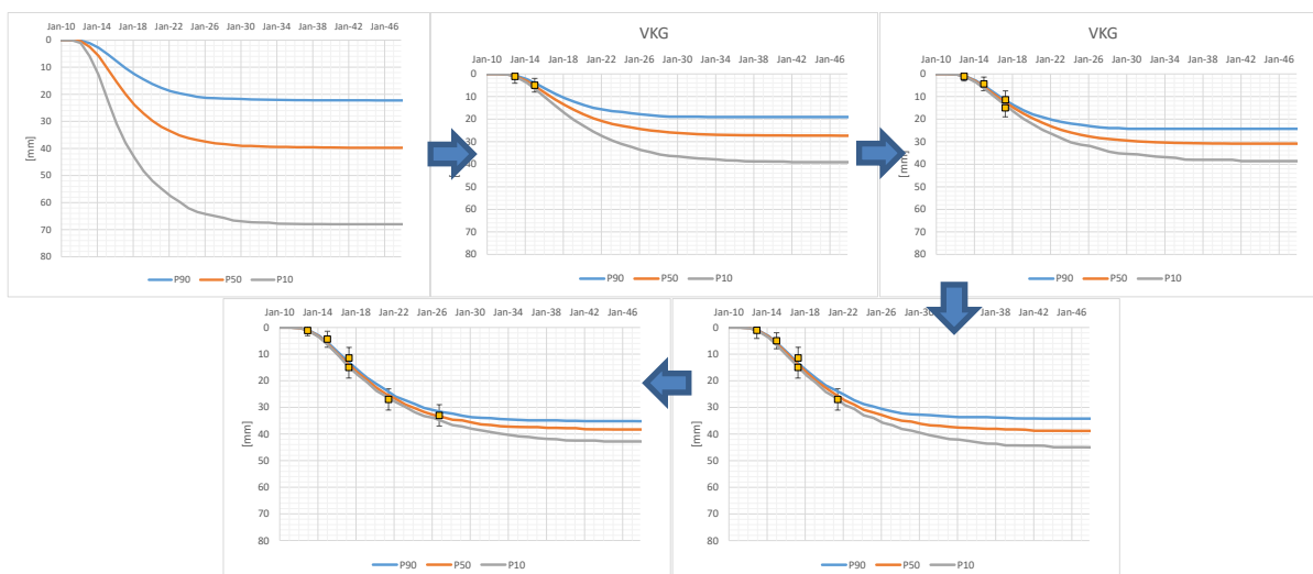
Figuur 2-15 Naarmate er meer metingen bijkomen, wordt de onzekerheid in de einddaling kleiner (rekenvoorbeeld). De verdeling voordat er metingen zijn (figuur linksboven) wordt de a priori verdeling genoemd.
