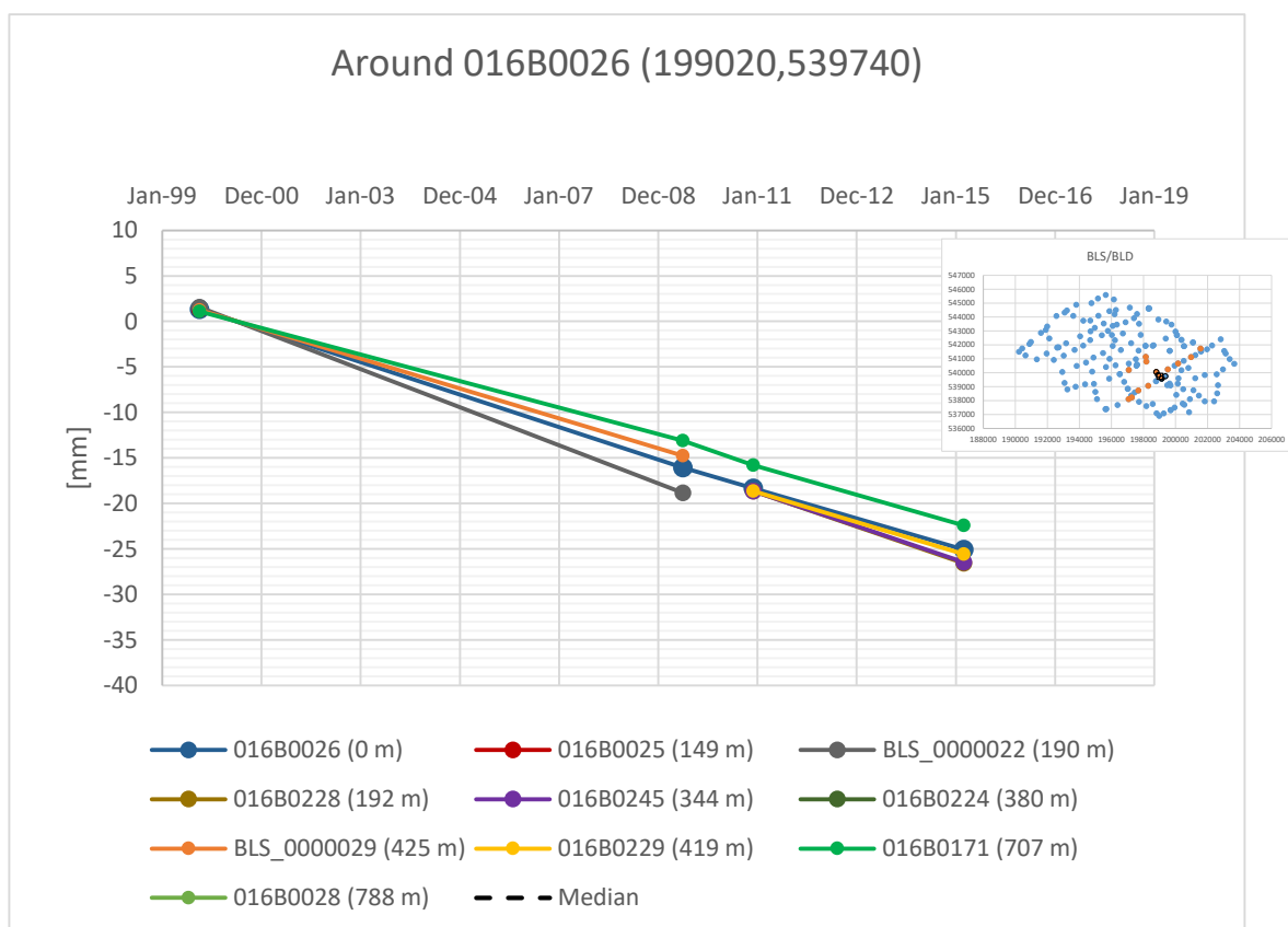
Figuur 15-1 Peilmerk daling rond het diepste punt van BLS. 1999-2009 is uit het meetplan BLS, 2010-2015 uit het meet plan BLD. De inzet geeft de locatie van de getoonde punten. (In de inzet zijn overlap-punten tussen de twee meetnetten oranje).
