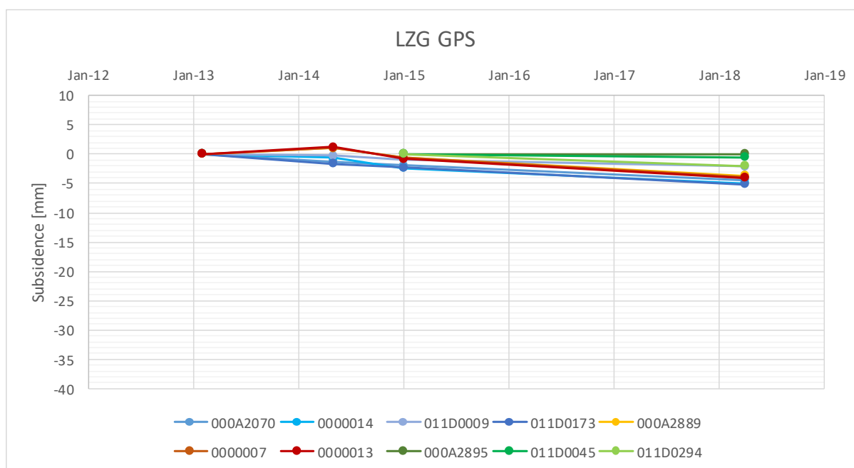
Figuur 13-1 Grafische weergave GPS-metingen. Een positieve waarde is een bodemstijging. Data uit ref. 44.
